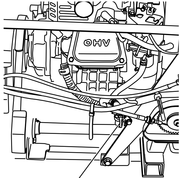
燃料コックレバー
